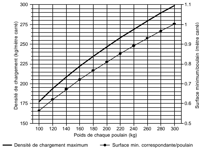
Densité de chargement max - Poulains Système métrique
