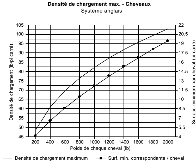
Figure 7 Espace minimum à allouer pour les chevaux libres durant le transport selon le poids corporel moyen individuel (syst. anglais). La ligne supérieure décrit la capacité de transport maximum de la remorque (axe de gauche); la ligne inférieure et l'axe de droite donnent l'espace minimum par animal. Une remorque standard de 102 po de largeur (largeur interne de 8,3 pieds) transportant des chevaux de 1 000 livres à raison de 76 lb/pi 2 transporterait 630 livres par pied de longueur du plancher. Les chevaux maigres ont besoin de plus d'espace que les chevaux en bon état de même poids. Réduisez la charge de 10 à 15 % dans des conditions chaudes et humides ainsi que pour les poulains transportés durant plus de 8 heures.
